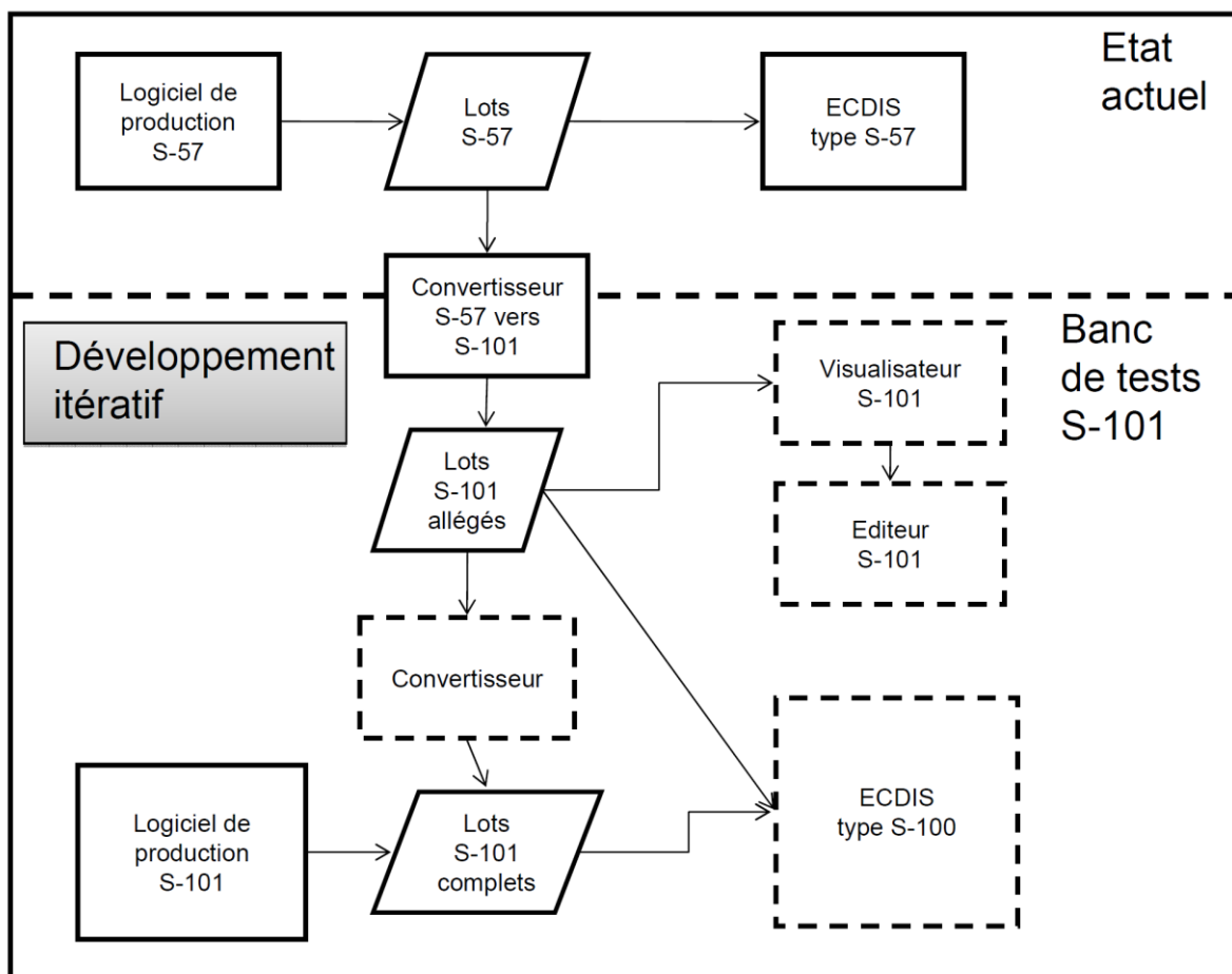
Figure 5: Banc d'essais de la norme S-101
